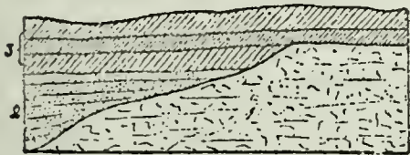
Fig. 3. Durchschnitt der Lager auf der nordöstlichen Seite der Klaas-Billenbay, in der unmittelbaren Nähe des grossen Gletschers (nach Dr. NATHORST). — 1. Krystallinische Schiefer. 2. Sandstein und kalkhaltiger Thonschiefer mit Pflanzenabdrücken. 3. Rother und weisser Gyps.
