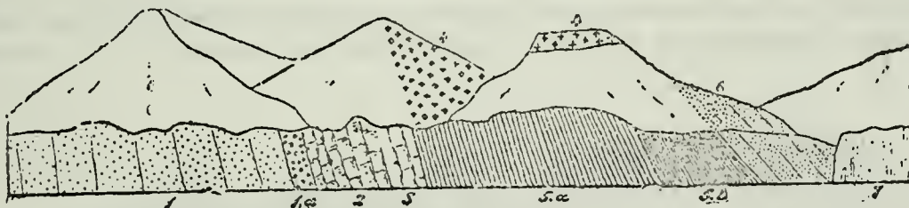
Fig. 4. Profil des nördlichen Strandes der Van Mijenbay, östlich vom Frithiofs-Gletscher.
