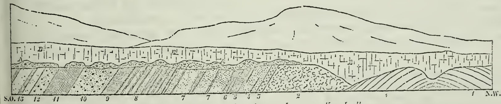
Fig. 17. Durchschnitt der miocenen Lager am Kap Lyell.
