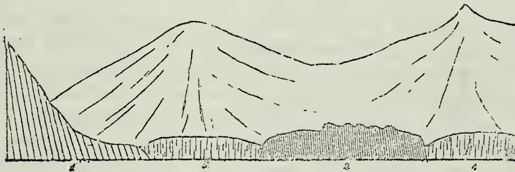
Fig. 6. Profil der Lager bei Safehaven.
