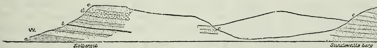
Fig. 16. Durchschnitt der tertiären Lager am nördlichen Ufer der van Mijenbay.
