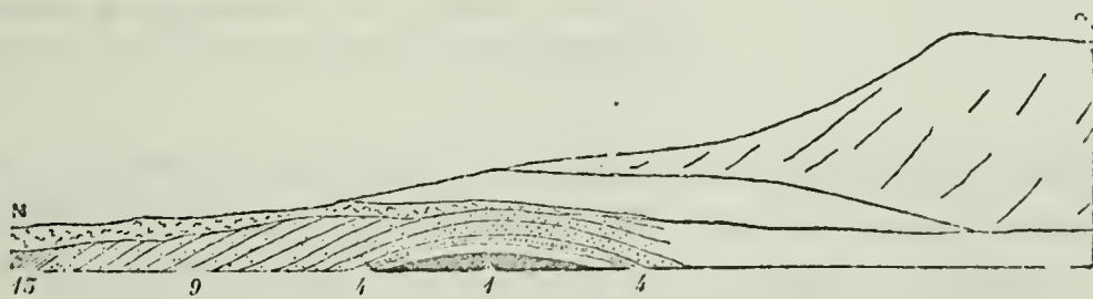
Fig. 15. Profil der Lager am Kap Heer.
