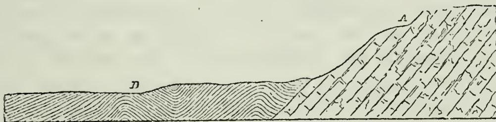
Fig. 19. Schematischer Durchschnitt, die Verwerfungen der tertiären Lager zeigend. A) Ältere Lager, der Bergkalk- oder Heklahookformation angehörend. B) Tertiäre Lager.
